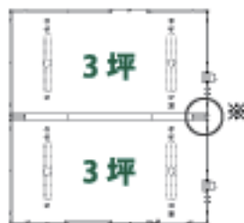
桁連棟 平面図
